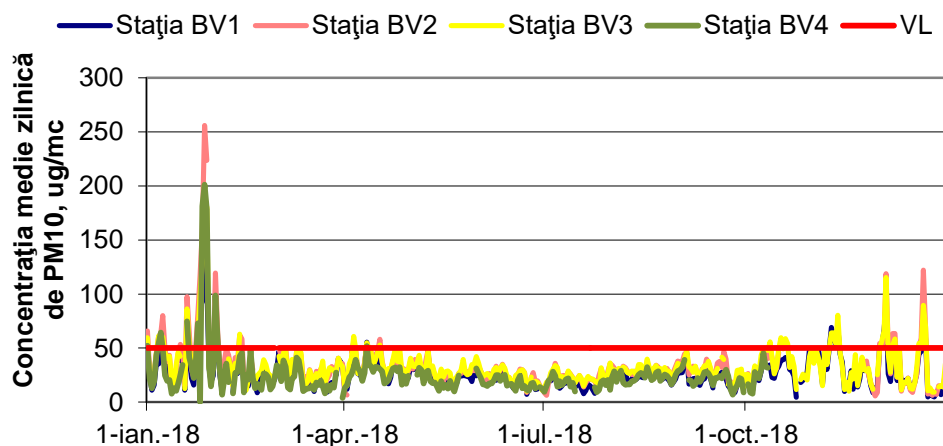
Figura 2: Evoluția mediilor zilnice de PM 10 în anul 2018
