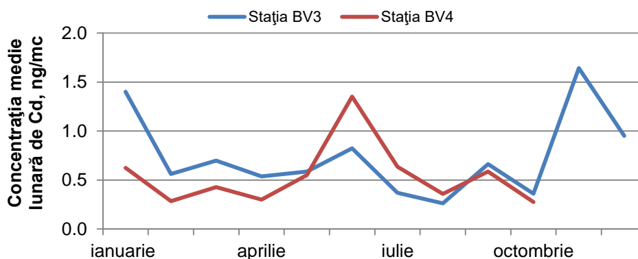
Figura 27: Evoluția mediilor lunare de cadmiu în anul 2018
