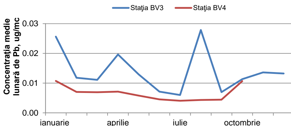
Figura 25: Evoluția mediilor lunare de plumb în anul 2018
