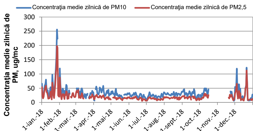
Figura 5 : Evoluția concentrației medii zilnice de PM 2,5 și PM 10 la stația BV2 în anul 2018
