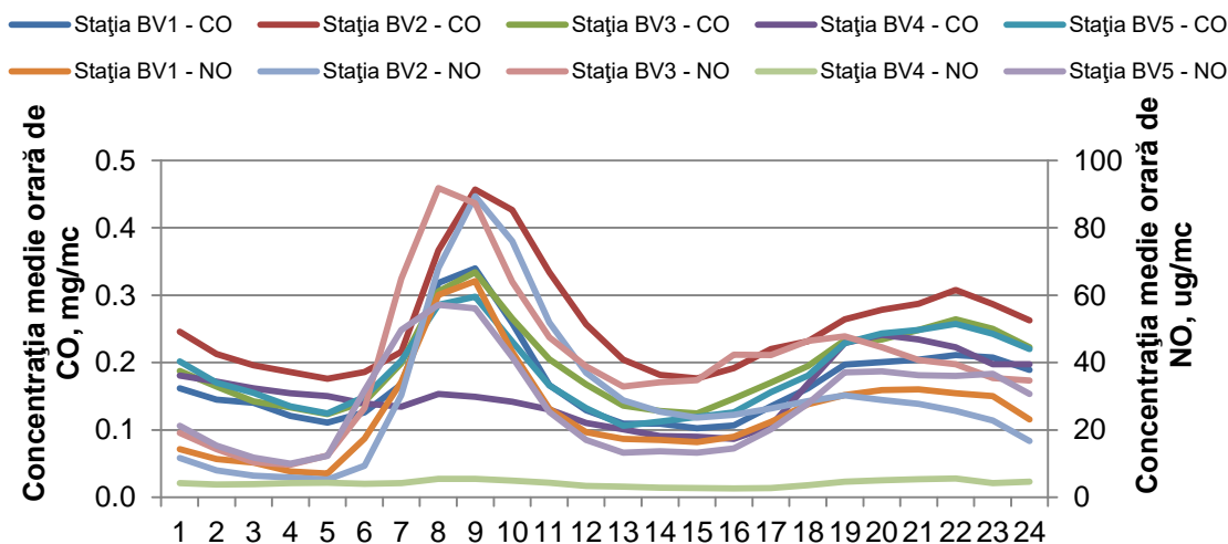
Figura 22: Ciclul zilnic al CO și NO
