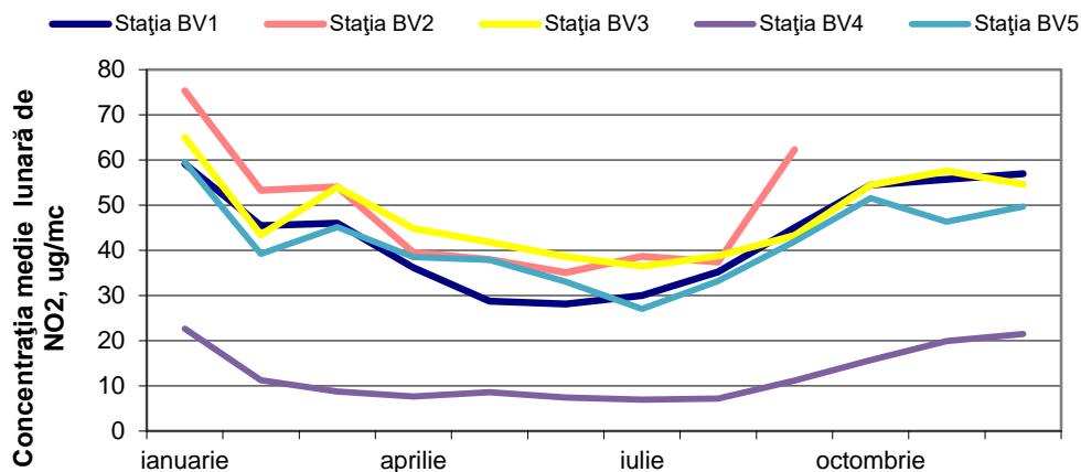
Figura 12: Evoluția concentrației medii lunare de NO 2 în anul 2018
