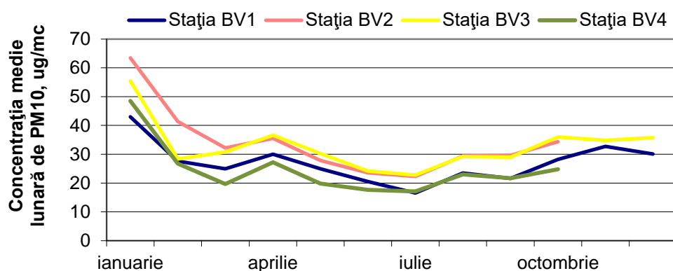
Figura 3: Evoluția mediilor lunare de PM10 în anul 2018
