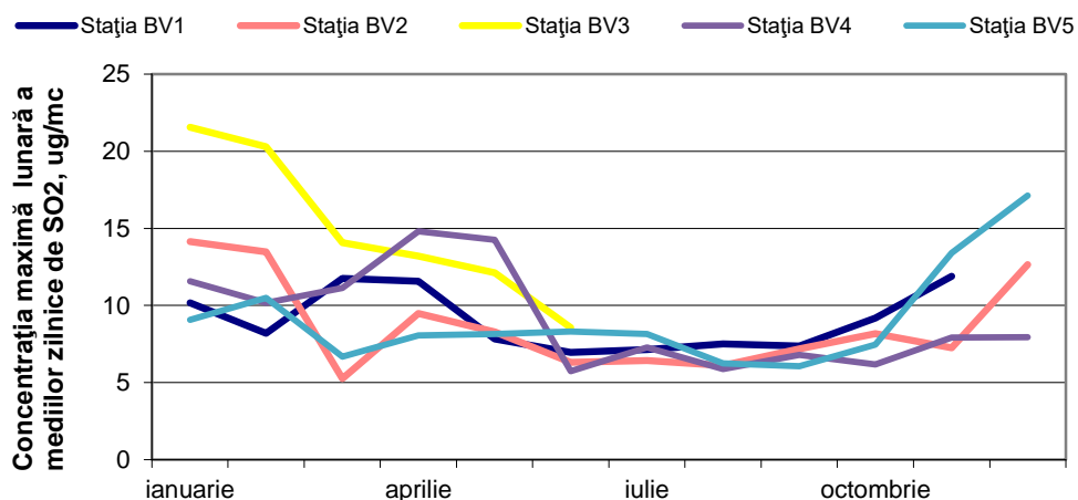
Figura 17: Evoluția maximelor lunare ale mediilor zilnice de \text{SO}_2 în anul 2018
