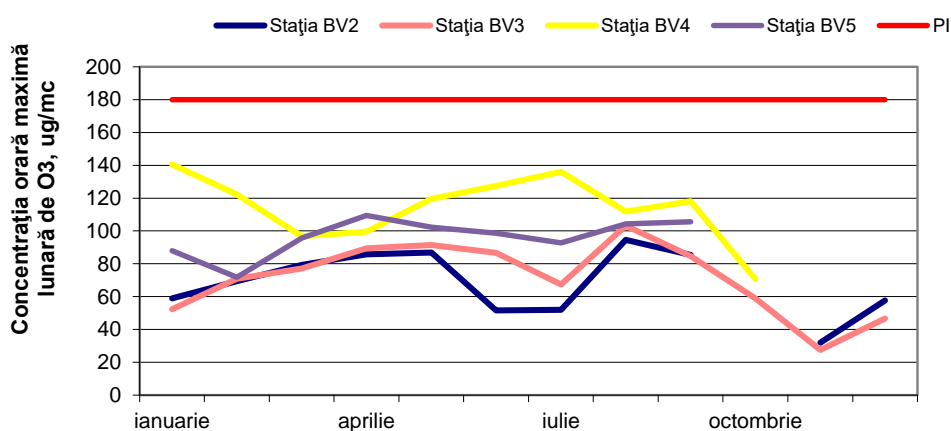
Figura 7: Evoluția maximelor lunare ale mediilor orare de O_3 în anul 2018
