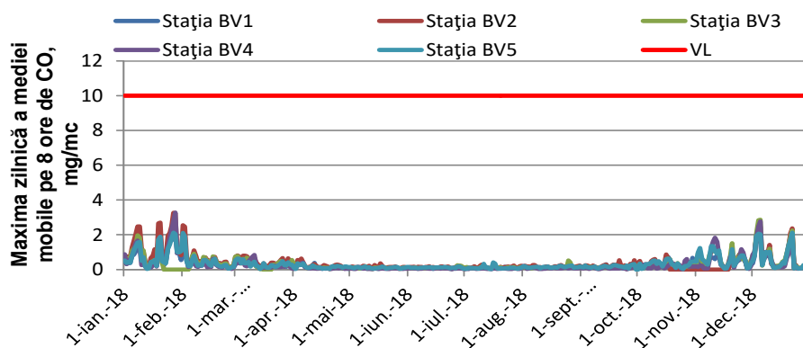
Figura 18: Evoluția valorilor maxime zilnice a mediilor mobile pe 8 ore de CO în anul 2018
