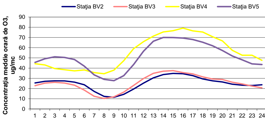
Figura 9: Ciclul zilnic al O 3
