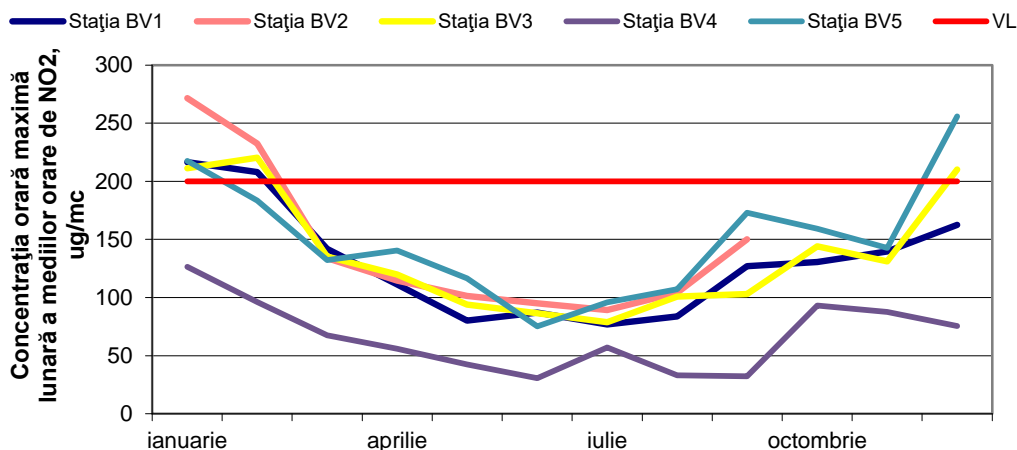
Figura 11: Evoluția concentrației maxime lunare a mediilor orare de NO 2 în anul 2018
