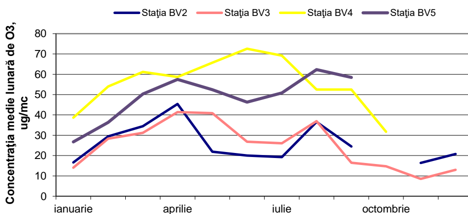
Figura 8: Evoluția mediilor lunare de O_3 în anul 2018
