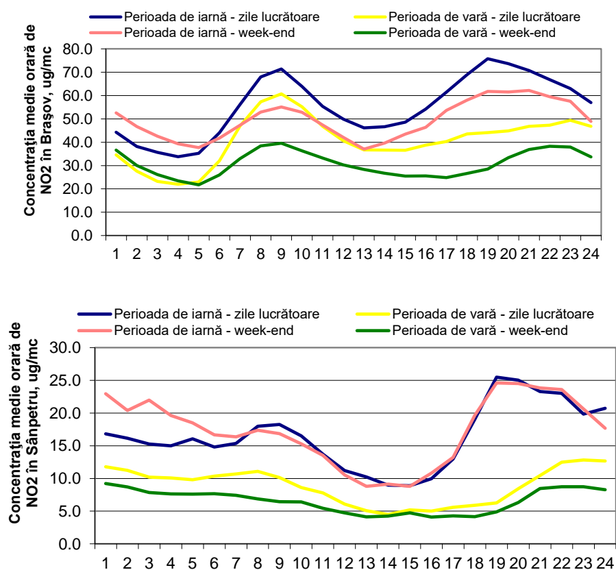
Figura 13: Ciclul zilnic al NO 2 în Brașov și Sânpetru
