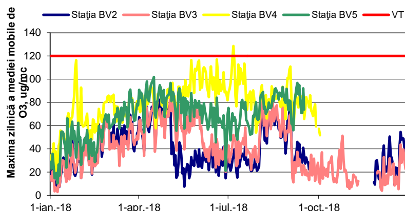
Figura 6: Evoluția maximelor zilnice ale mediilor mobile pe 8 ore de O 3
