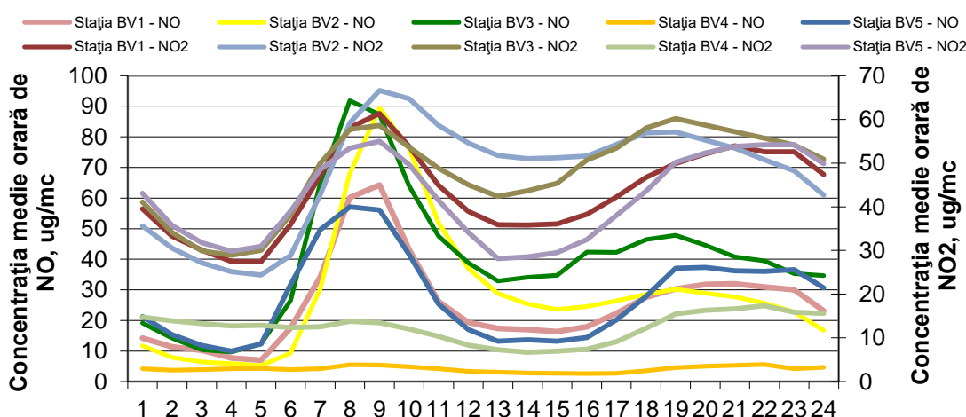
Figura 15: Ciclul zilnic al NO 2 și NO
