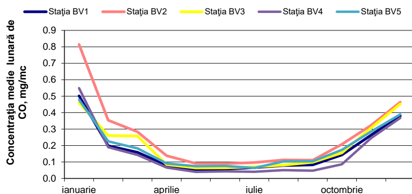
Figura 19: Evoluția mediilor lunare de CO în anul 2018
