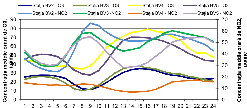
Figura 10: Ciclul zilnic al O 3 și NO 2
