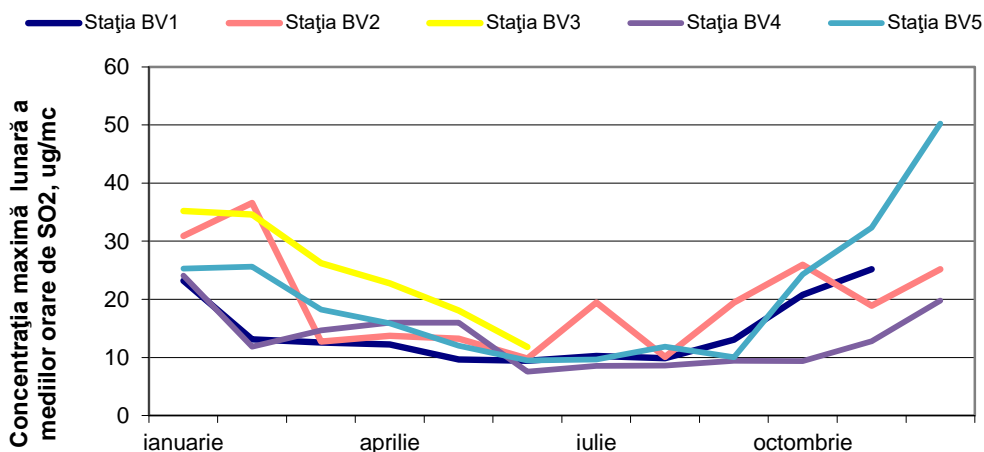
Figura 16: Evoluția maximelor lunare ale mediilor orare de SO 2 în anul 2018
