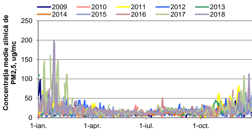
Figura 4: Evoluția mediilor zilnice de PM 2,5
