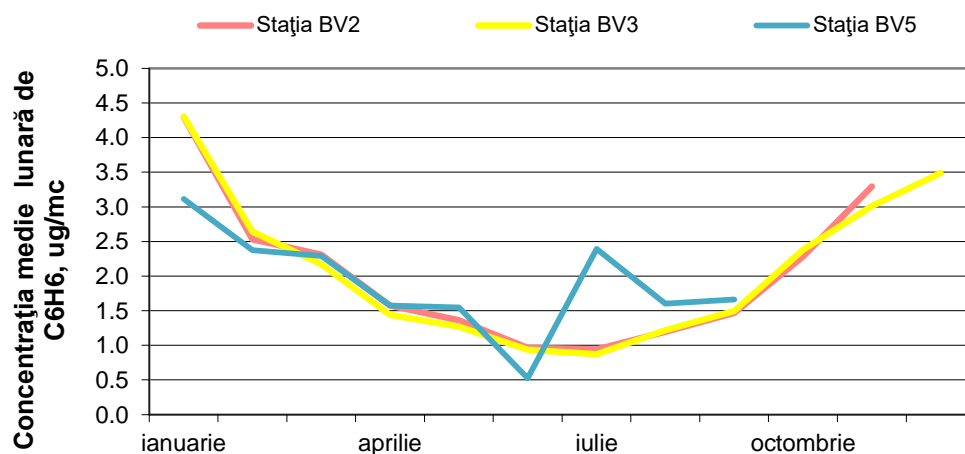
Figura 23: Evoluția mediilor lunare de benzen în anul 2018
