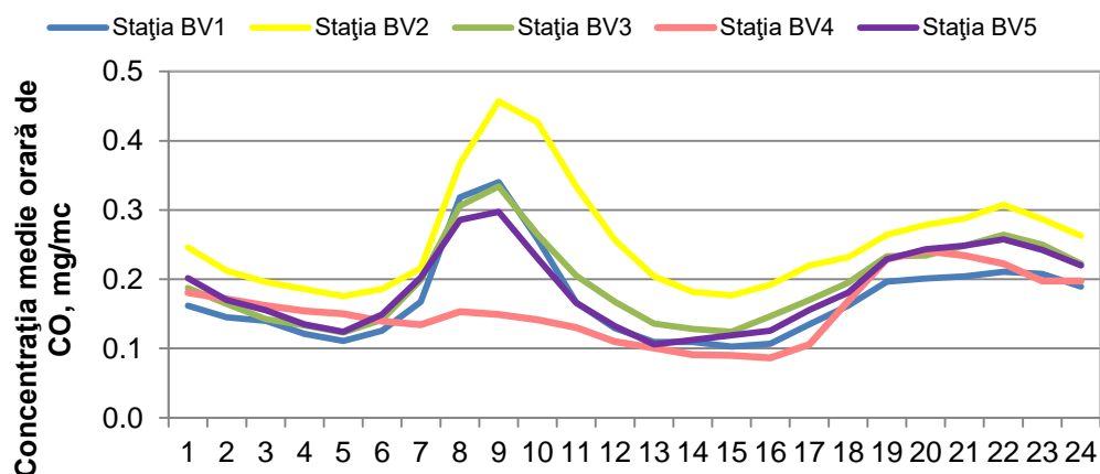
Figura 21: Ciclul zilnic al CO în timpul săptămânii și anului
