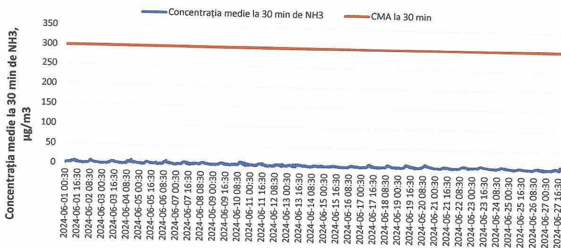
Figura 8. Evoluția concentrațiilor medii la 30 min. de amoniac în luna iunie 2024
