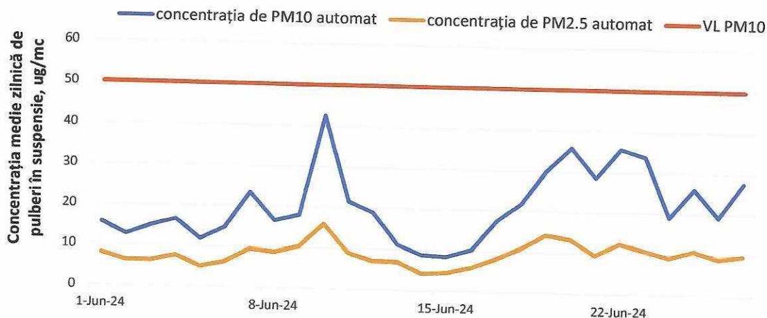
Figura 7. Evoluția concentrațiilor medii zilnice de PM10 (automat) în luna iunie 2024
