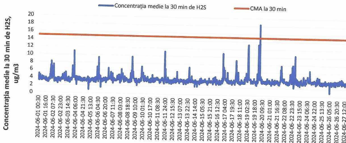
Figura 10. Evoluția concentrațiilor medii la 30 min. de hidrogen sulfurat în luna iunie 2024
