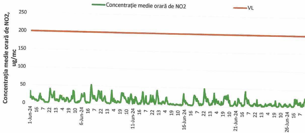
Figura 2. Evoluția concentrațiilor medii orare de NO 2 în luna iunie 2024
