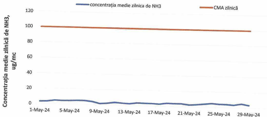
Figura 9. Evoluția concentrațiilor zilnice de amoniac în luna mai 2024
