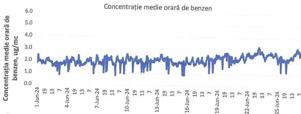
Figura 6. Evoluția concentrațiilor medii orare de benzen în luna iunie 2024
