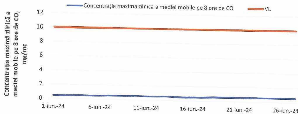
Figura 5. Evoluția maximelor zilnice ale mediei mobile de CO în luna iunie 2024
