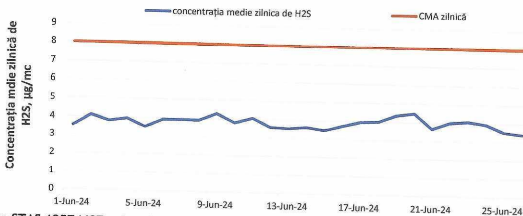
Figura 11. Evoluția concentrațiilor zilnice de H 2 S în luna iunie 2024
