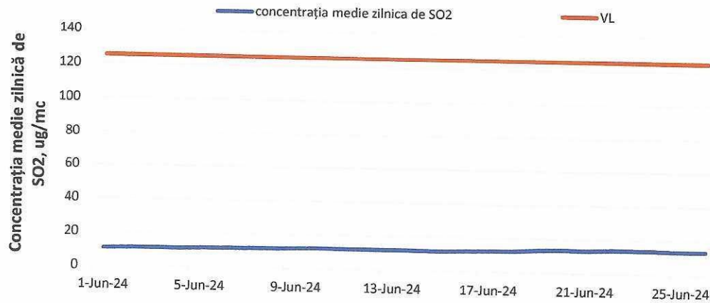
Figura 4. Evoluția concentrațiilor medii zilnice de SO 2 în luna iunie 2024
