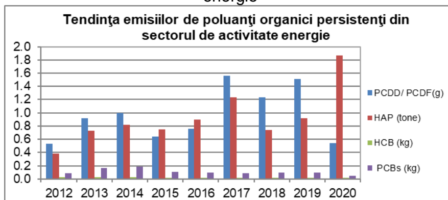
Figura 1.68: Tendința emisiilor de poluanți organici persistenți din sectorul de activitate energie
