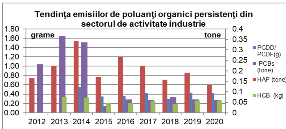
Figura 1.69: Tendința emisiilor de poluanți organici persistenți din sectorul de activitate industrie
