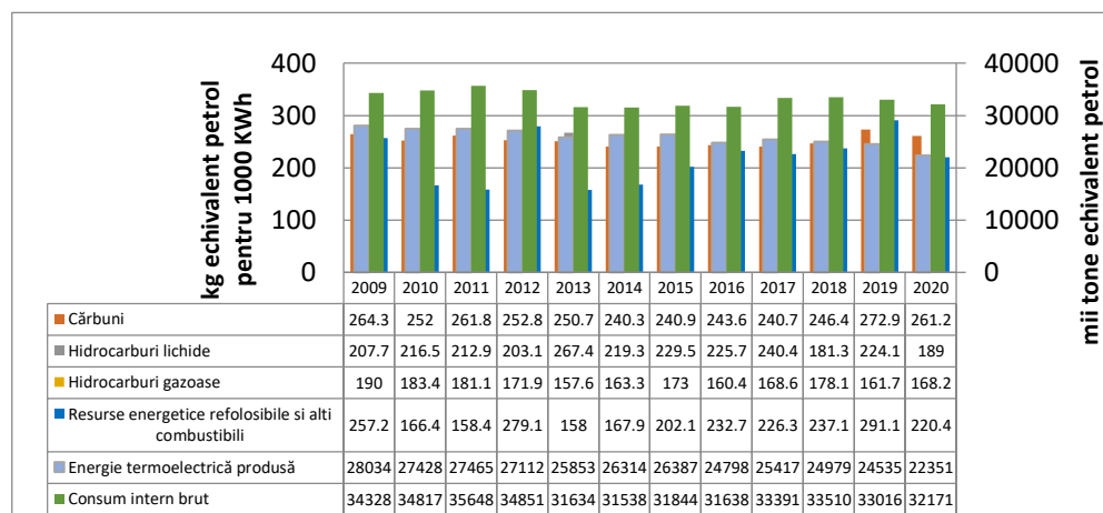
Figura I.31: Consumul specific de combustibil pentru producerea energiei termoelectrice la nivel național
