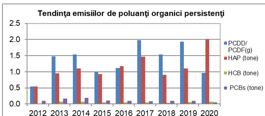
Figura 1.67: Tendința emisiilor de poluanți organici persistenți
