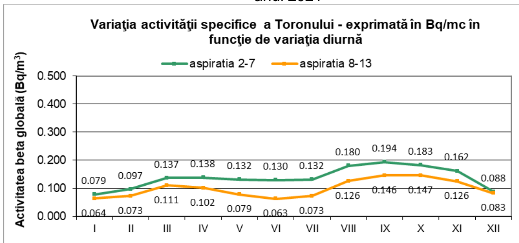
Figura IX.6. Variația activității specifice medii lunare a toronului din atmosferă în anul 2021
