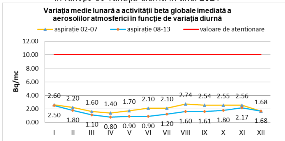
Figura IX.2. Variația medie lunară a activității beta globale imediate a aerosolilor atmosferici în funcție de variația diurnă în anul 2021
