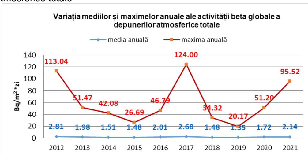
Figura IX.10. Variația mediilor și maximelor anuale ale activității beta globale a depunerilor atmosferice totale
