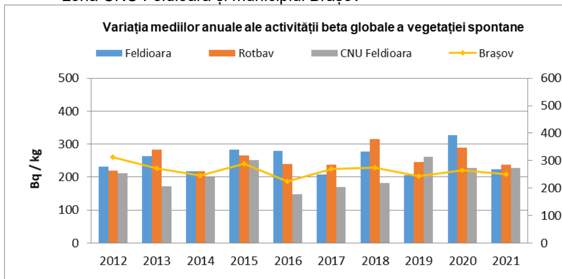
Figura IX.17. Variația mediilor anuale ale activității beta globale a vegetației spontane din zona CNU Feldioara și municipiul Brașov
