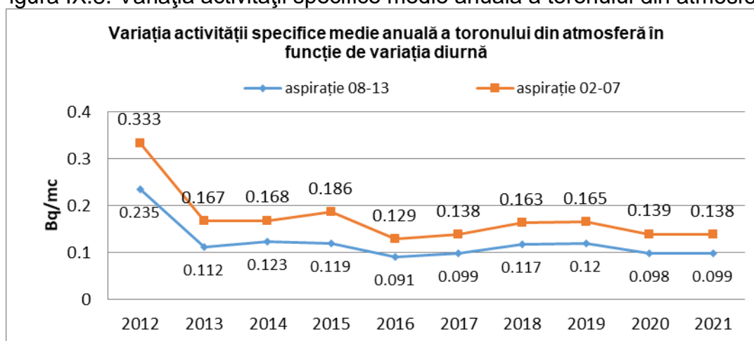
Figura IX.8. Variația activității specifice medie anuală a toronului din atmosferă
