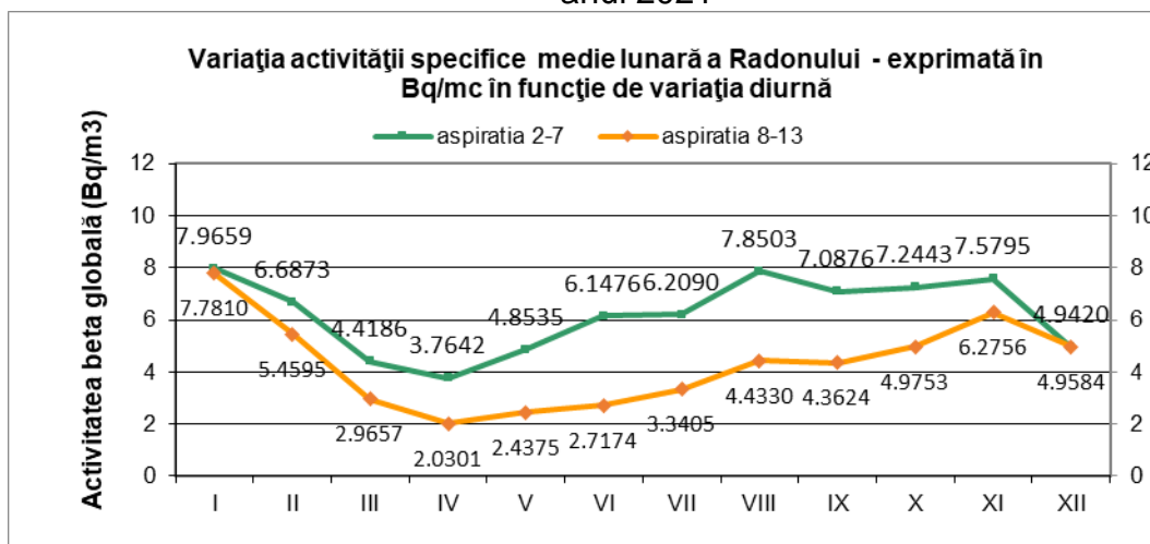
Figura IX.5. Variația activității specifice medii lunare a radonului din atmosferă în anul 2021
