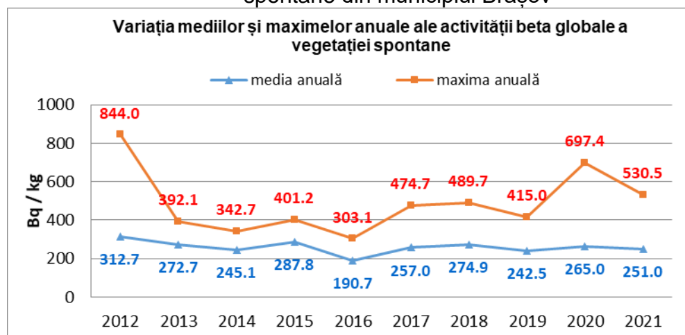
Figura IX.16. Variația mediilor și maximelor anuale a activității beta globale a vegetației spontane din municipiul Brașov
