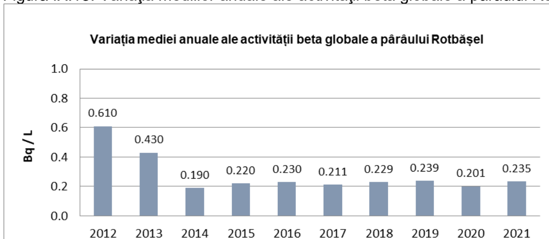
Figura IX.13. Variația mediilor anuale ale activității beta globale a pârâului Rotbășel
