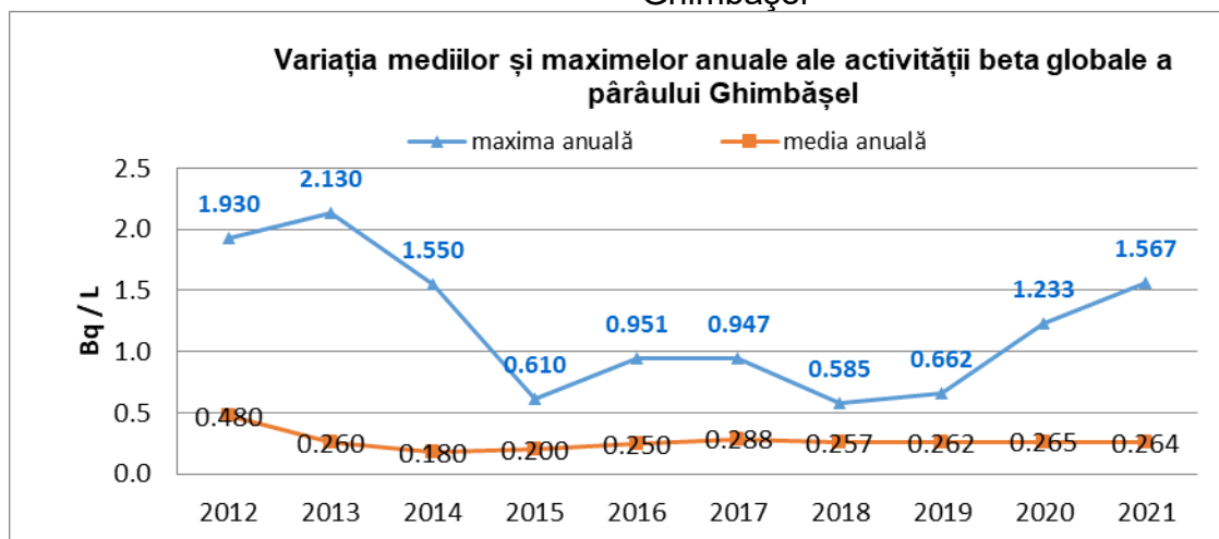
Figura IX.11. Variația mediilor și maximelor anuale ale activității beta globale a pârâului Ghimbășel
